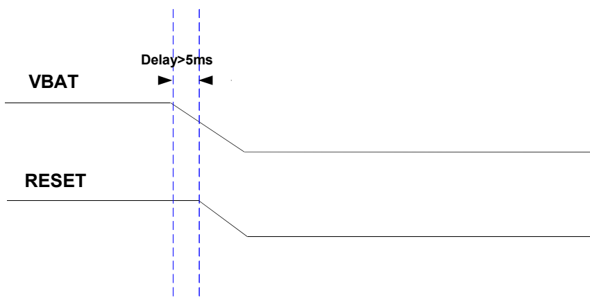
图 5：关机时序
