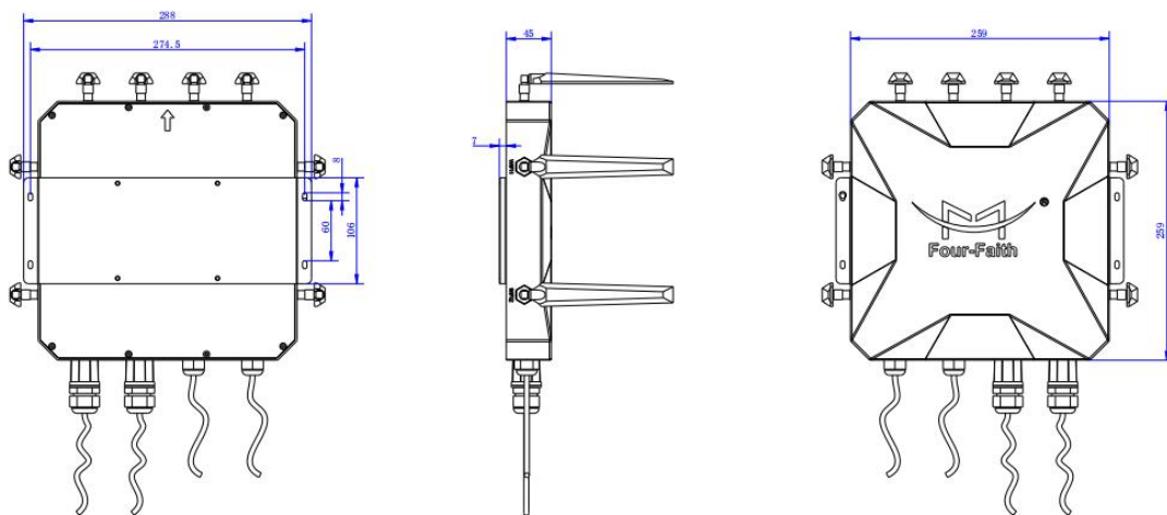
挂壁安装方式 (标配)
