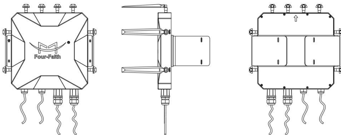
抱杆安装方式 (选配)
