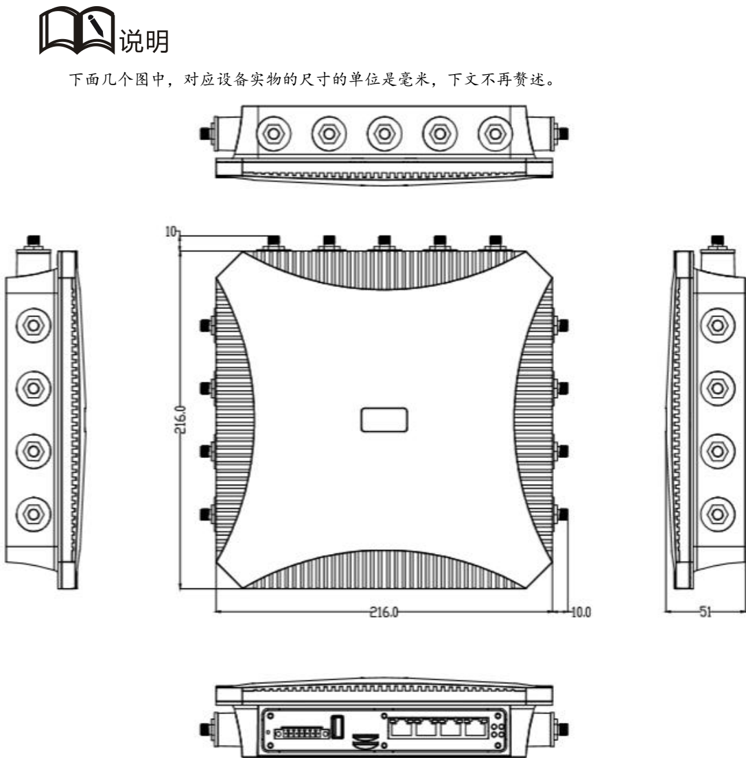
图 2-2 Z1 工业智能网关结构尺寸图
