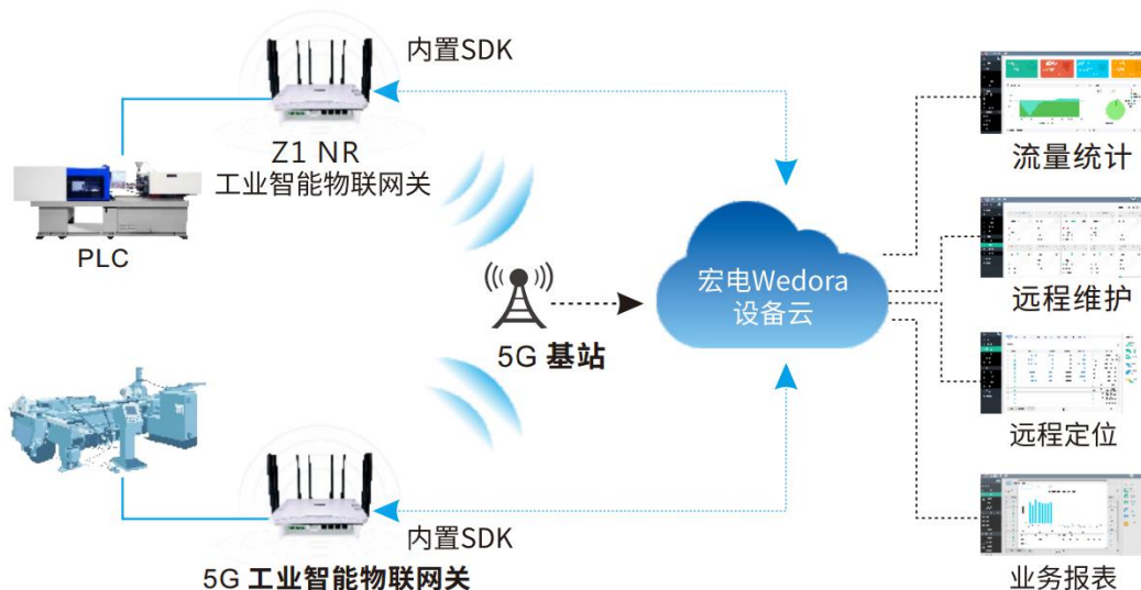
图 1-1 智能工厂设备无线联网应用示意图
