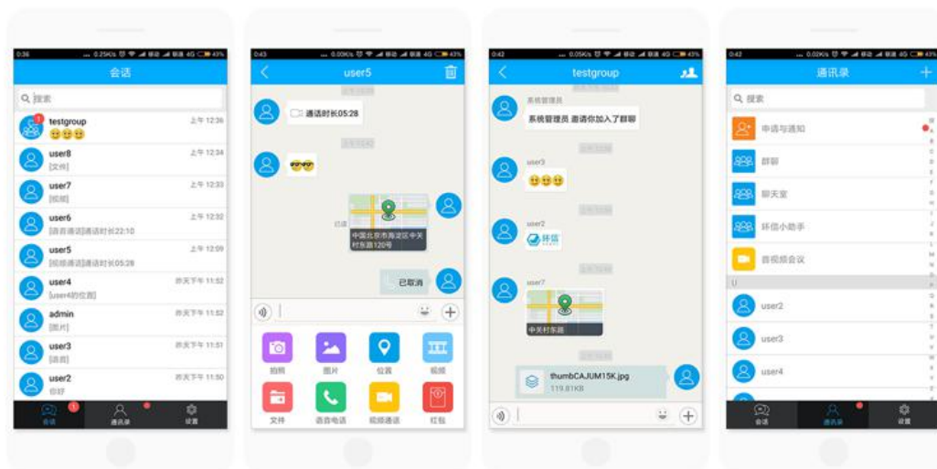
会话列表
