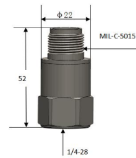
外形示意图
