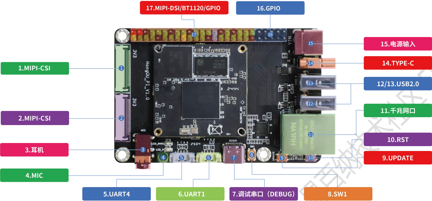
正面接口图
