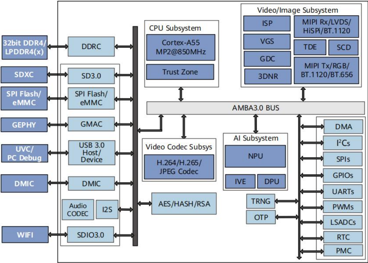
Hi3516DV500 功能框图
