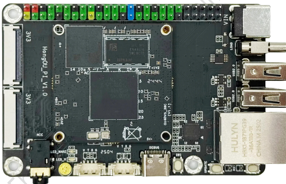
产品外观图
