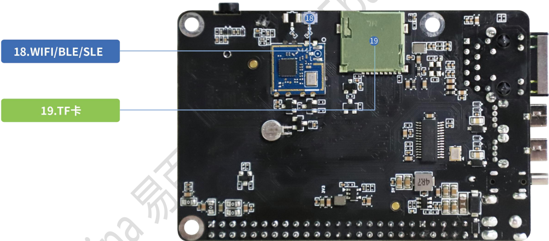
反面接口图
