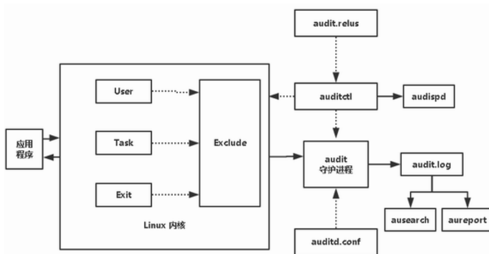
图 8-10 架构示意图
