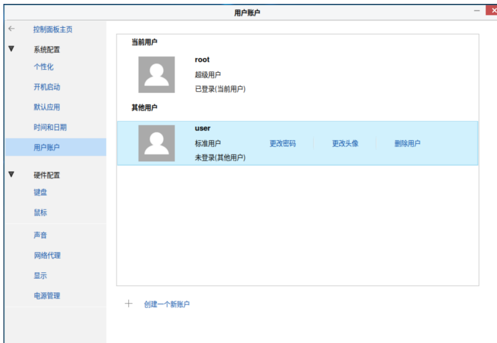
图 1-2 用户账户
