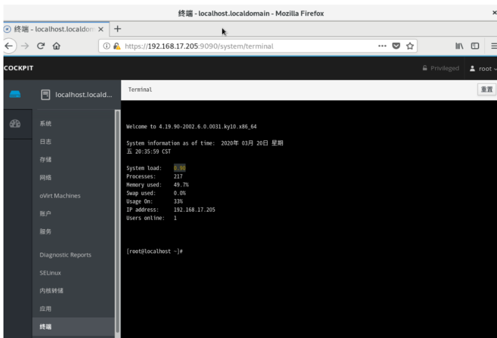
图 3-26 终端界面
