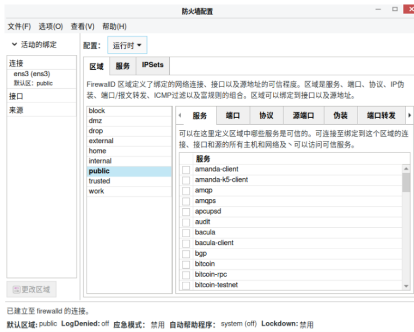
图 8-1 防火墙配置
