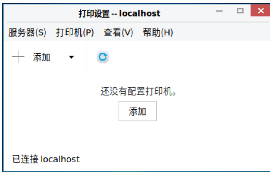
图 6-1 打印设置
