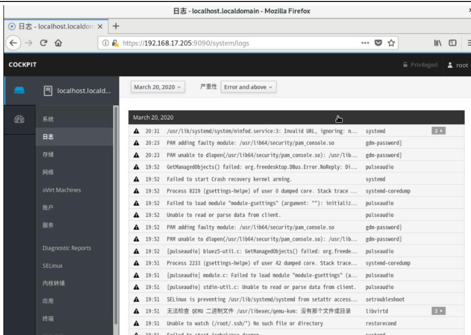
图 3-23 日志界面
