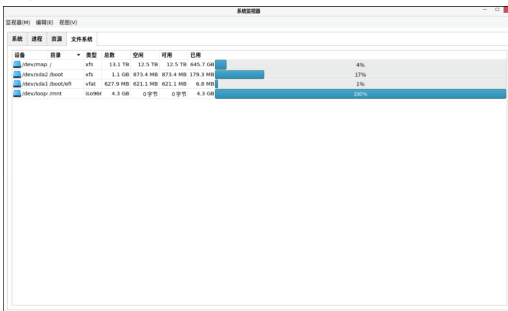
图 7-3 文件系统
