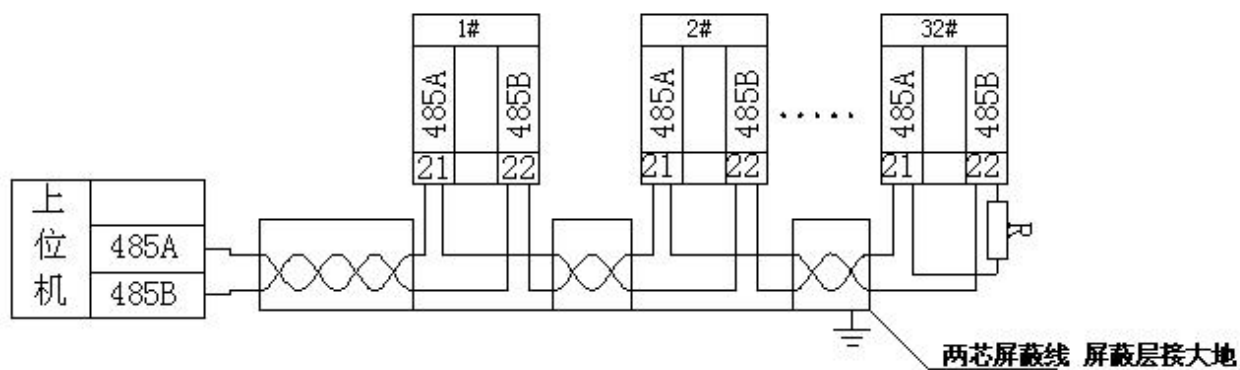
图 10 RS485 通讯接线示意图 建议最末端仪表的 A、B 之间加匹配电阻，阻值范围为 120\Omega \sim 10\text{ k}\Omega 。
