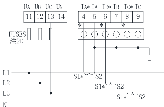
3P3L/3CT (仪表设置为3P4L) 注②
