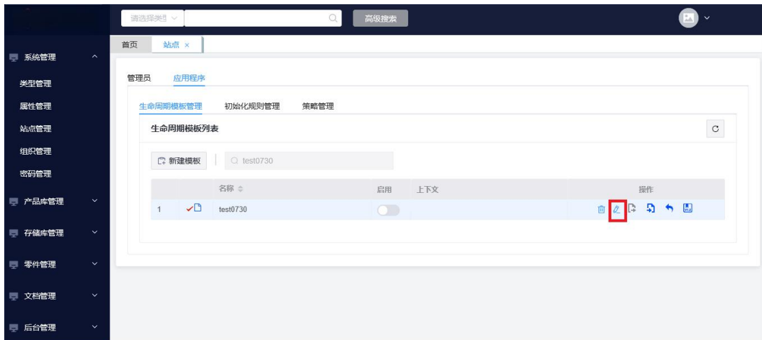
图 34 检出
