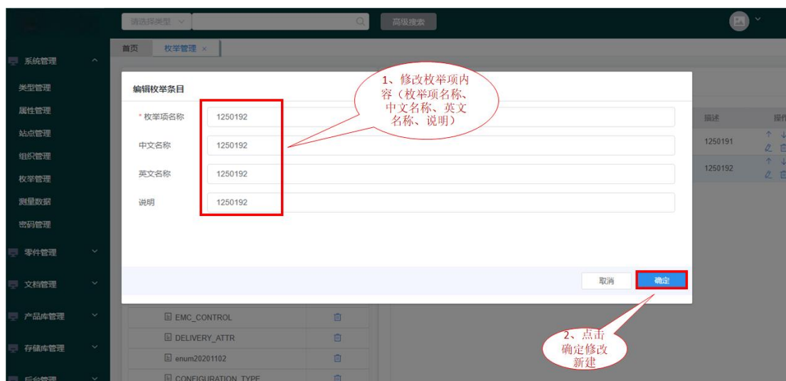
图 26 修改枚举项
