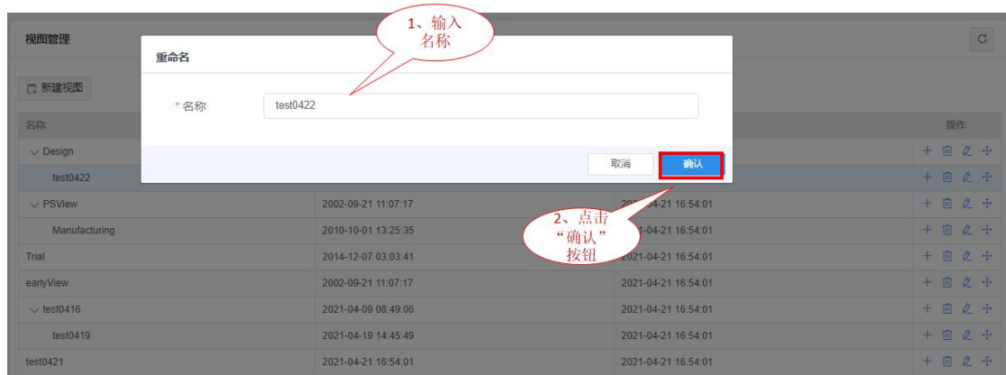
图 54 重命名视图
