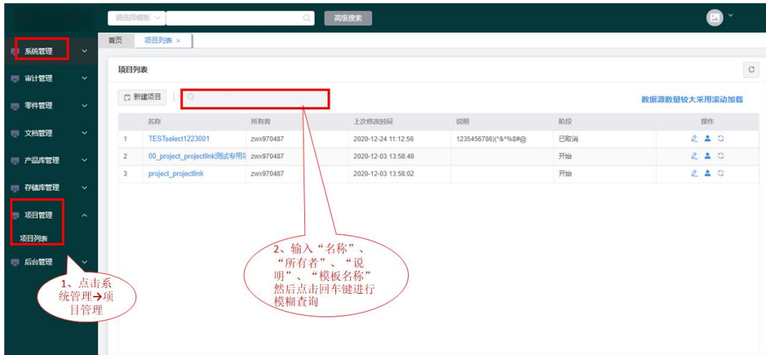
图 19 查询项目
