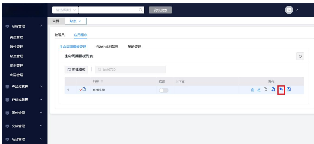
图 35 撤销检出
