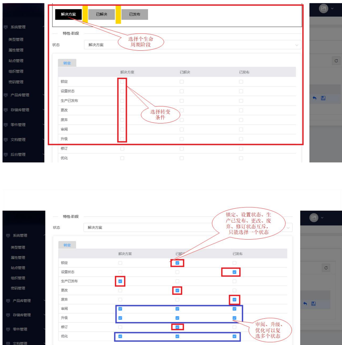
图 39 参与者管理
