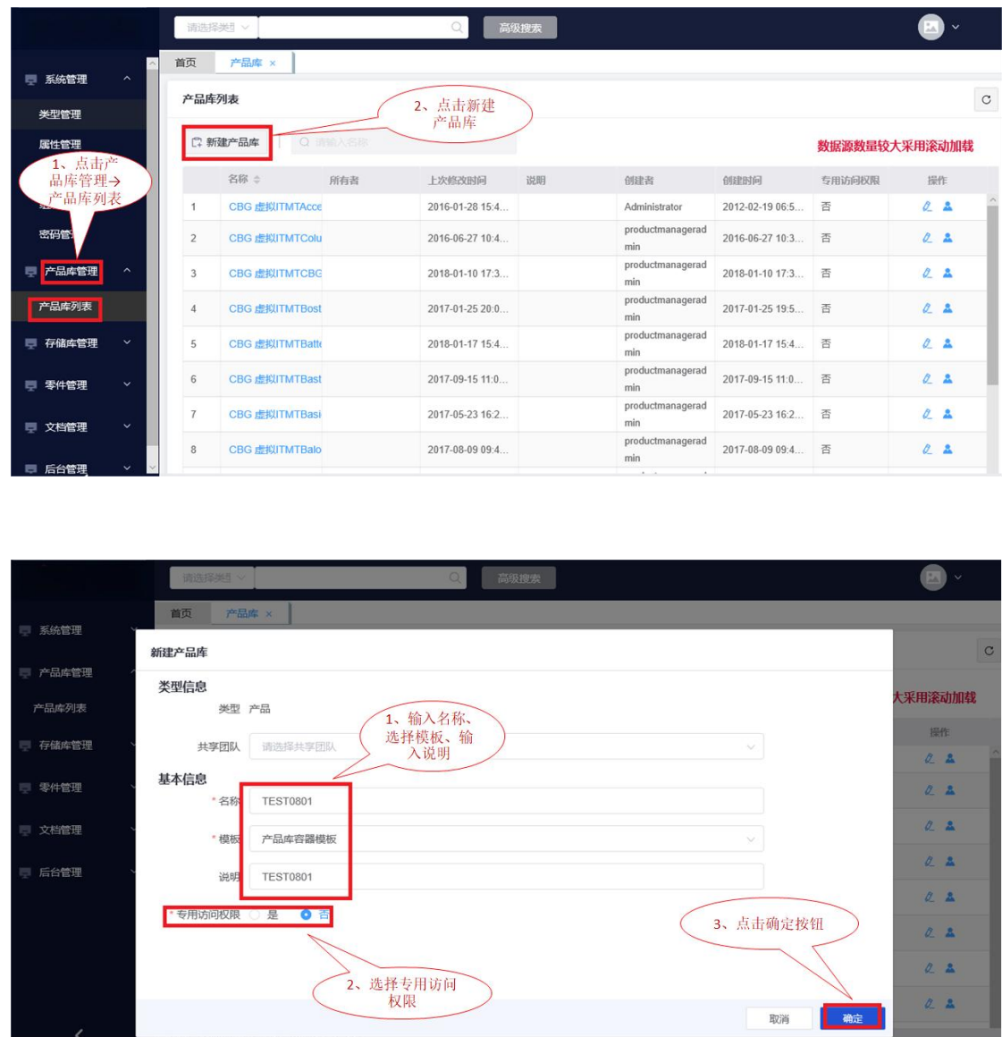
图 3 新建产品库
