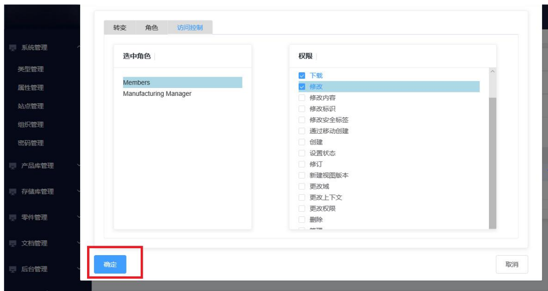
图 41 定义权限
