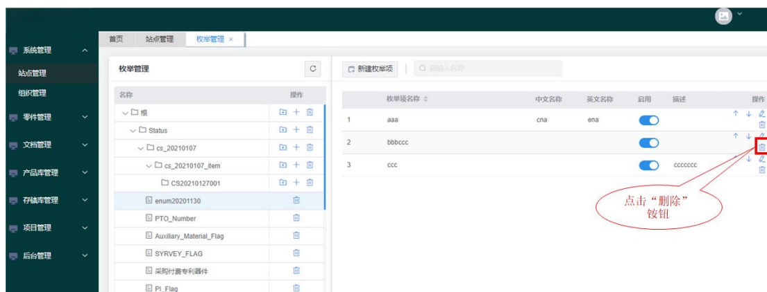
图 27 删除枚举项
