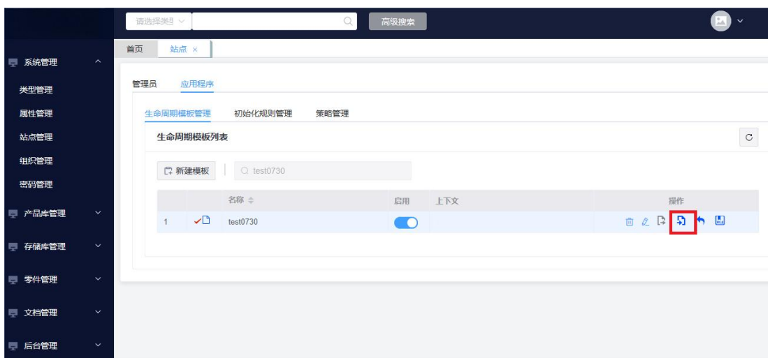
图 36 检入
