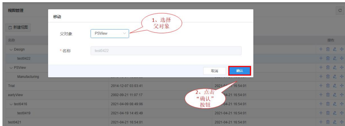
图 55 移动视图
