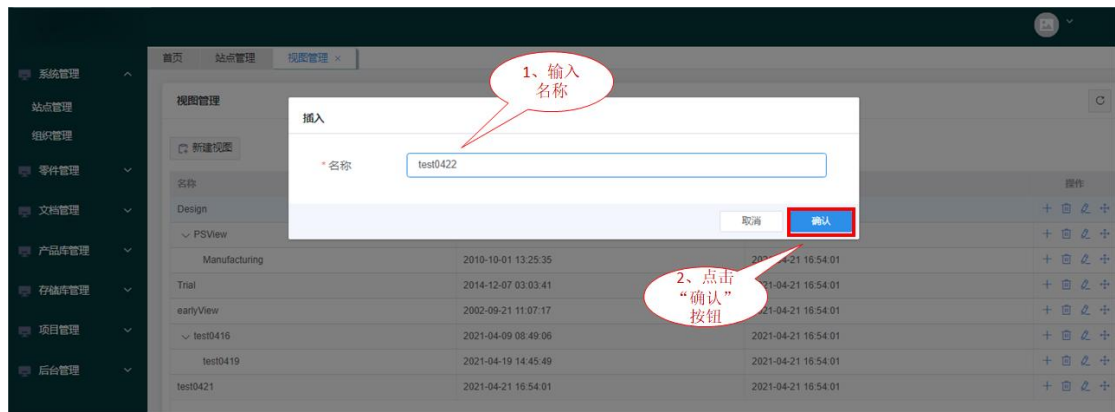
图 53 插入视图
