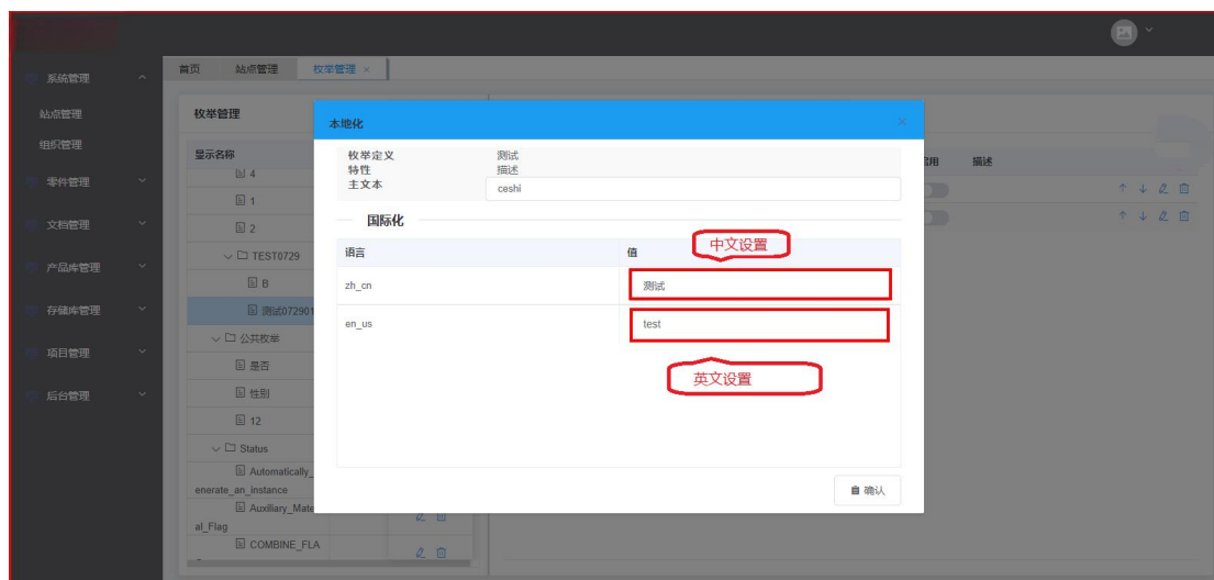
图 29 枚举多语言
