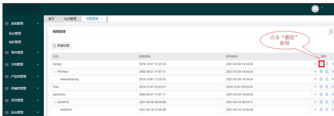
图 56 删除视图
