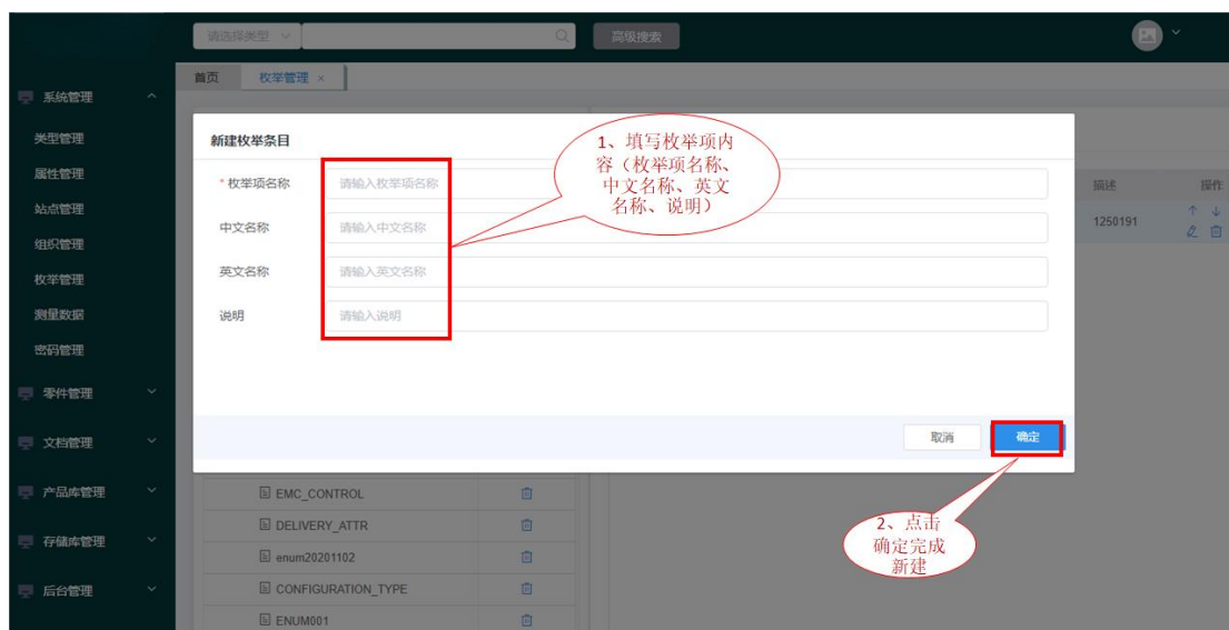
图 25 新建枚举项
