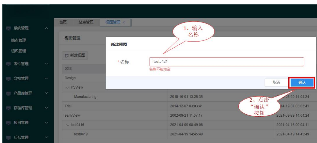
图 52 新建视图
