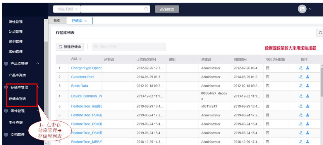
图 16 存储库
