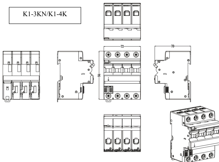
图 6: K1-3KN、K1-4K 智慧微断产品示意图
