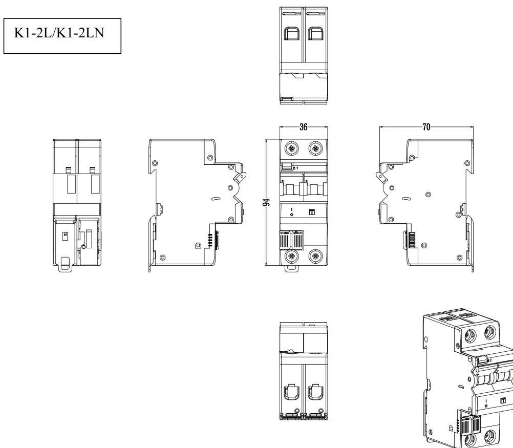
图 7: K1-2L 智慧微断产品示意图
