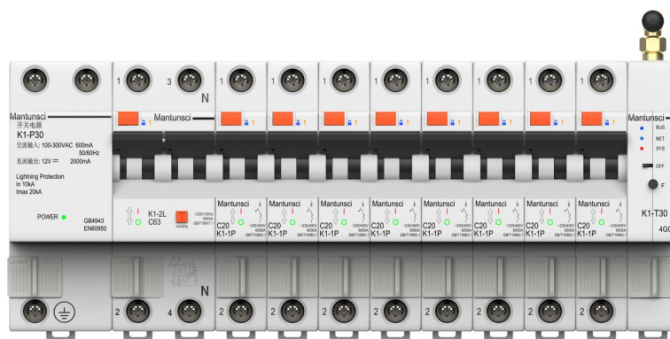
图 14：智慧微断产品连接完成示意图
