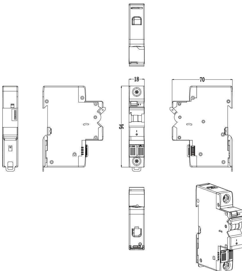
图 1: K1-1P 智慧微断产品示意图
