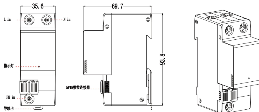
图 10：K1 系列智慧微断匹配智能电源模组示意图
