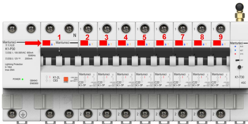
图 16 设置地址图示说明
