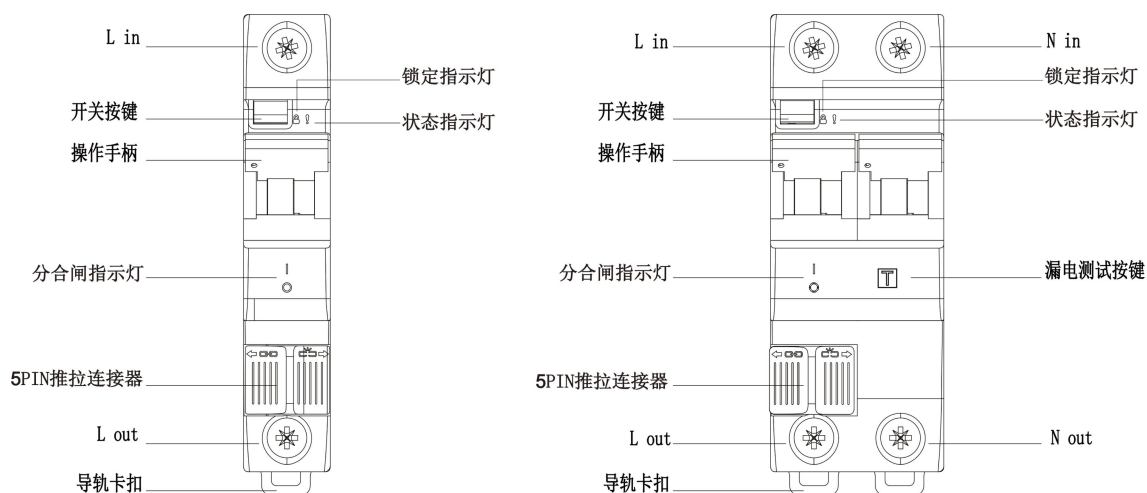
图 13: 智慧微断模组功能示意图
