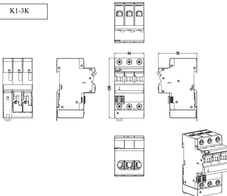
图 5: K1-3K 智慧微断产品示意图
