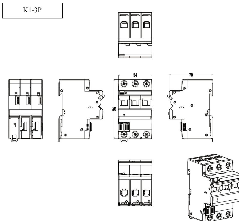
图 3: K1-3P 智慧微断产品示意图
