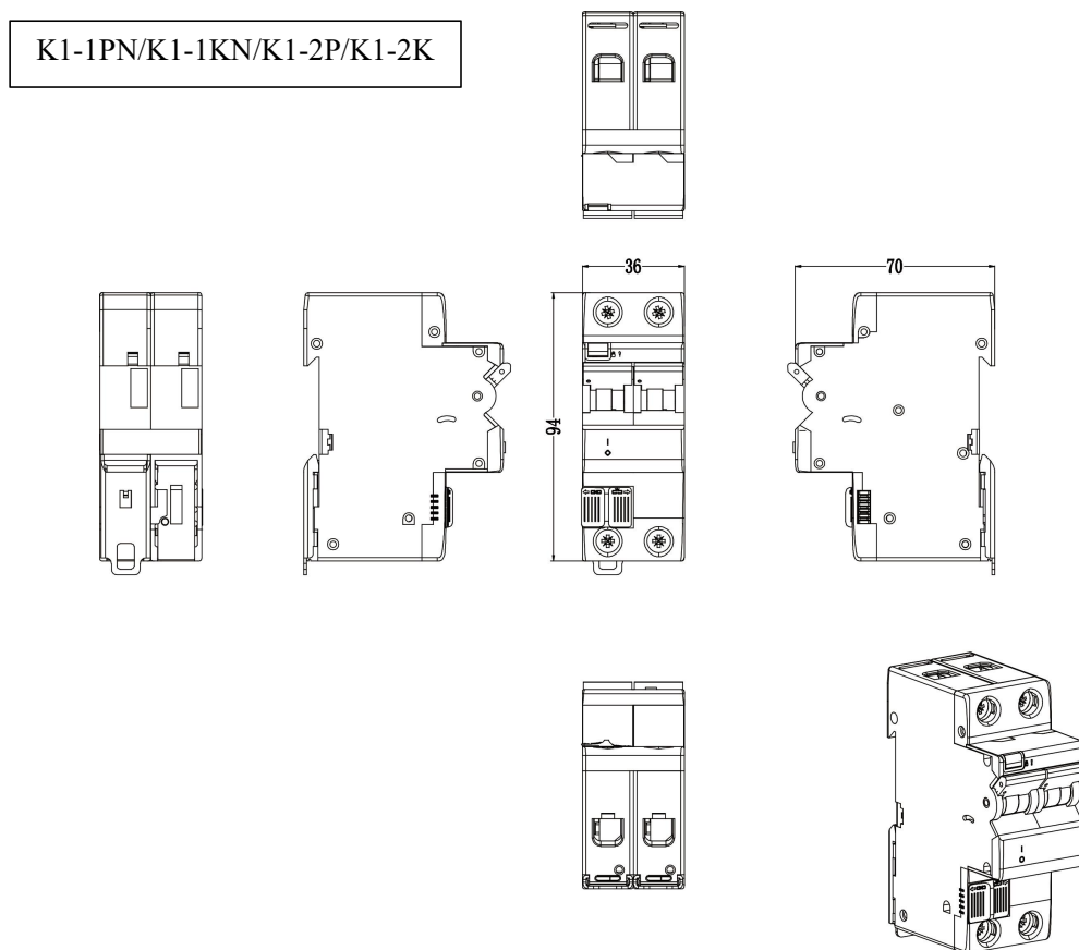
图 2: K1-1PN/K1-1KN/K1-2P/K1-2K 智慧微断产品示意图
