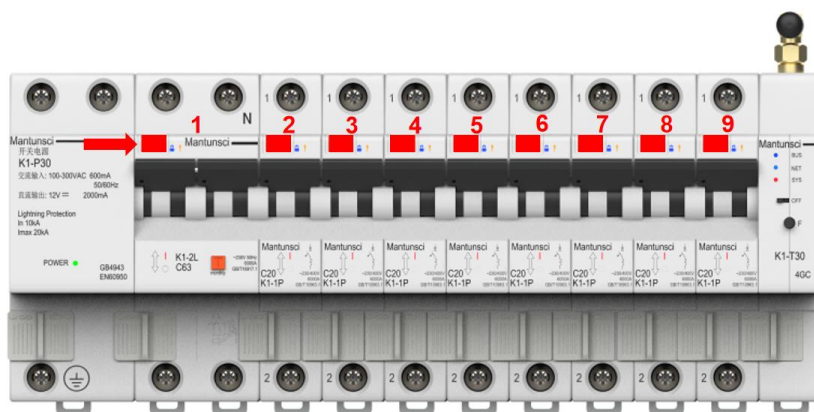
图 15 设置地址图示说明
