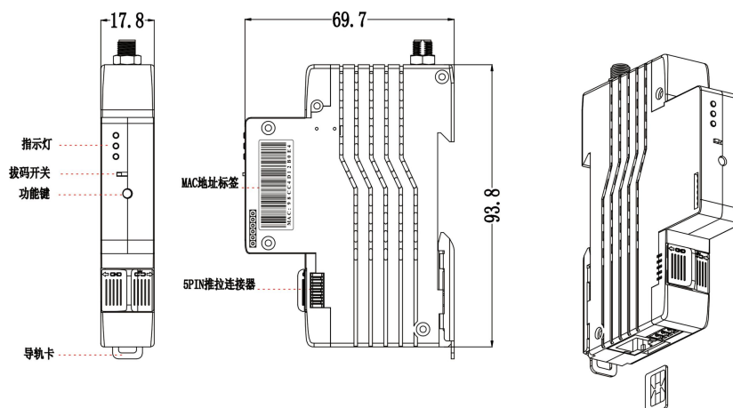
图 11：K1 系列智慧微断匹配通讯模组示意图
