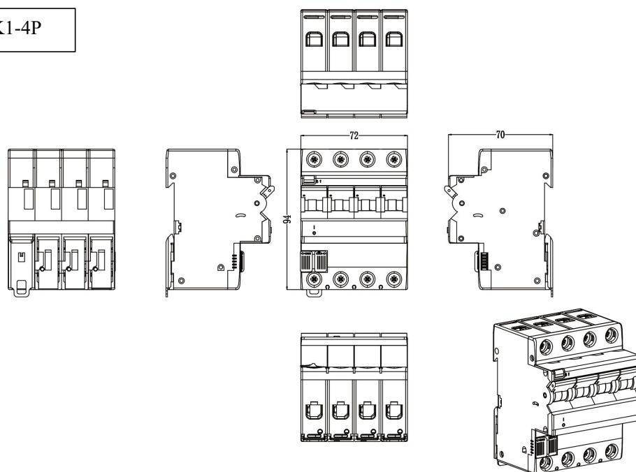
图 4: K1-3PN、K1-4P 智慧微断产品示意图
