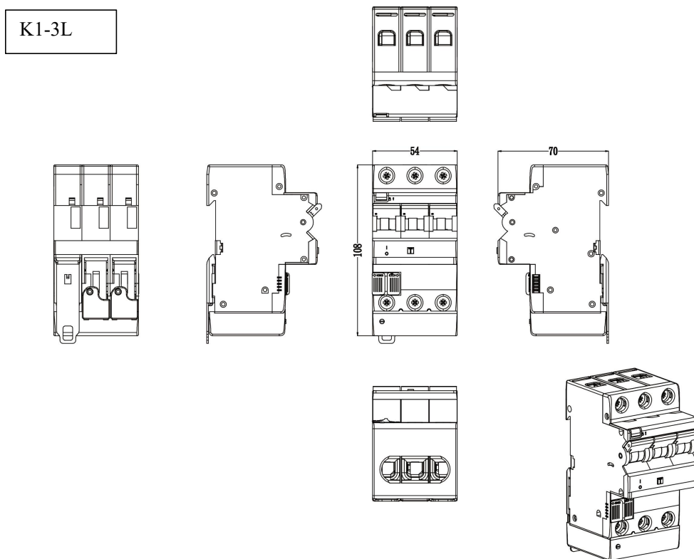
图 8: K1-3L 智慧微断产品示意图
