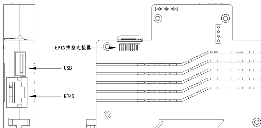
图 12: K1 系列智慧微断匹配边缘计算模组示意图
