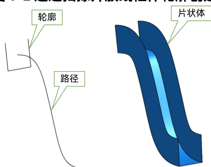
图 7-1 通过扫掠开放线框体轮廓创建片状体
