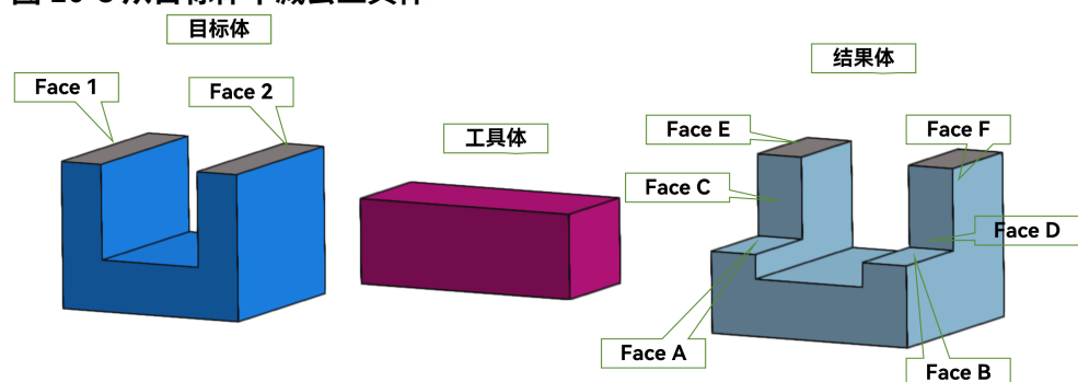
图 10-8 从目标体中减去工具体
