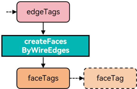
图 2-10 调用函数将面附着到线框体
