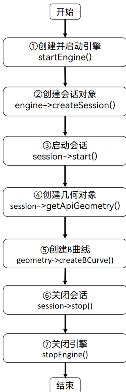
图 4-1 接口调用流程图
