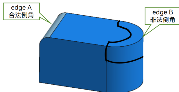
图 12-8 非法倒角阻止全面检查的示例
