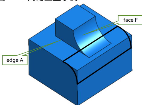
图 12-6 倒角重叠示例
