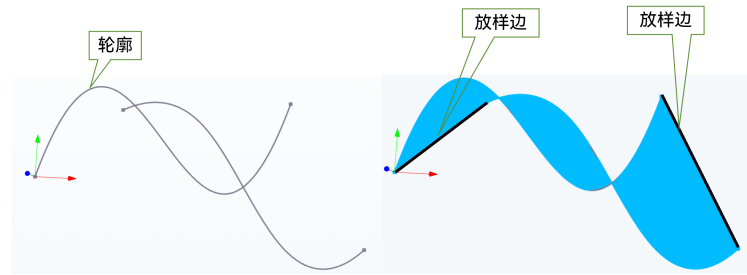
图 7-11 由两个共面轮廓创建的自交片状体
