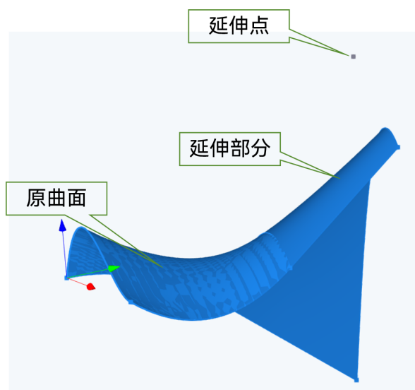
图 8-6 延伸到一个指定的顶点
