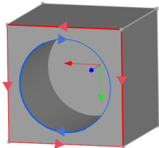
图 3-6 一个面上的外环与内环
