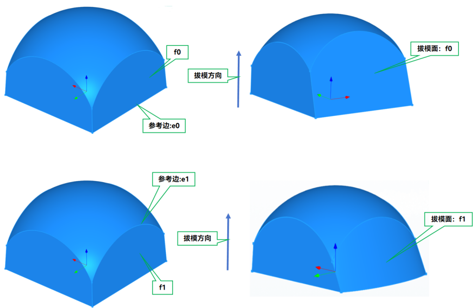
图 6-4 选择 e0 和 e1 做为参考实体
