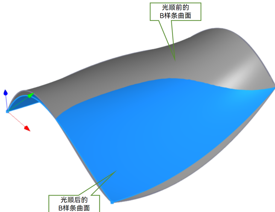
图 6-9 光顺普通 B 样条曲面示例
