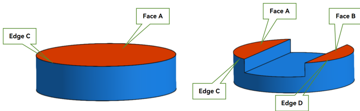
图 10-7 两个面共享同一个曲面
