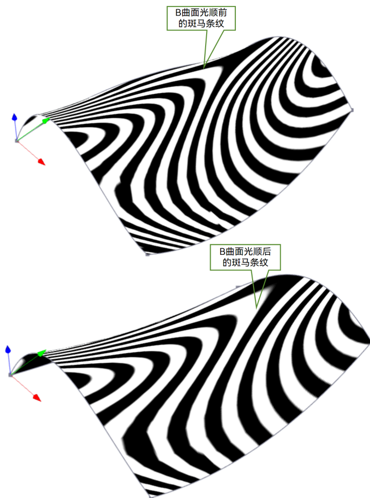
图 6-10 光顺普通 B 样条曲面
