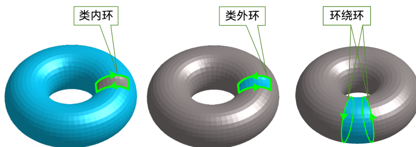
图 3-9 圆环面中的环
