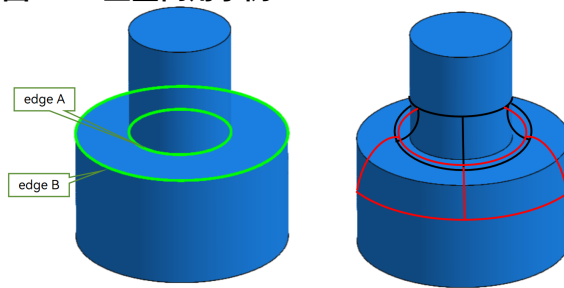
图 12-9 重叠倒角示例
