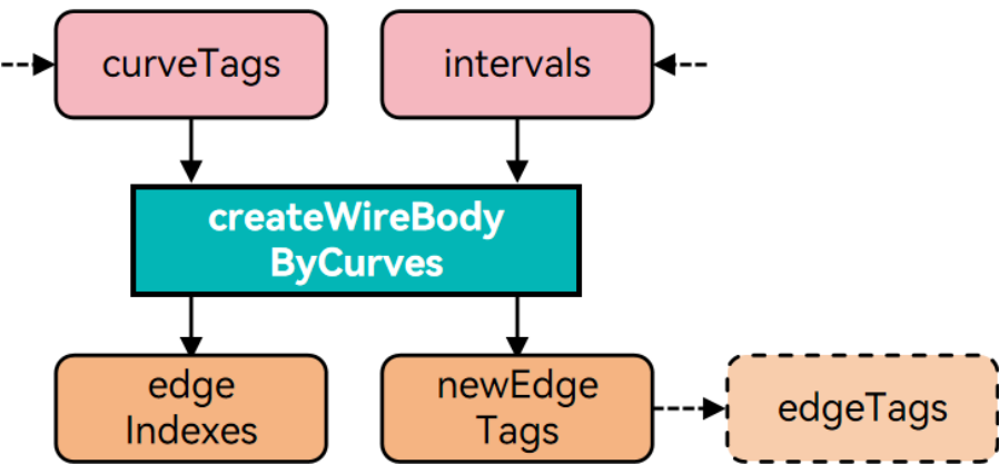
图 2-8 调用函数创建线框体
