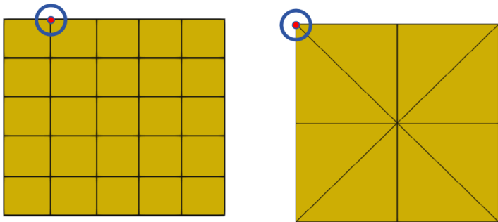
图 3-21 开放片状体中的顶点（一个面集，一条普通边和两个边界边）
