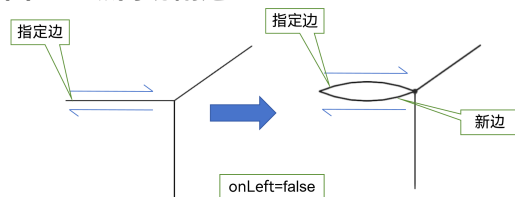
图 9-2 纵向切割边
