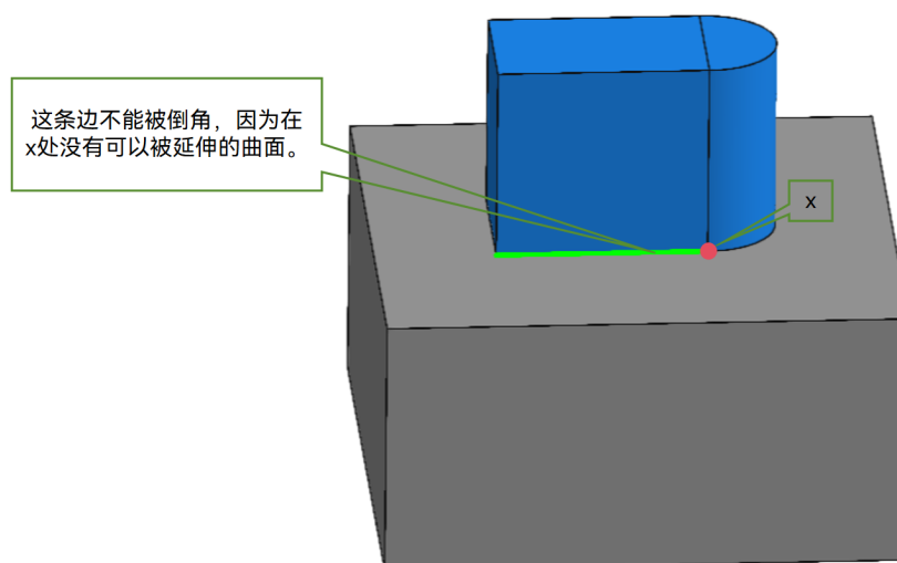
图 12-3 在一个顶点上倒角一条边的限制
