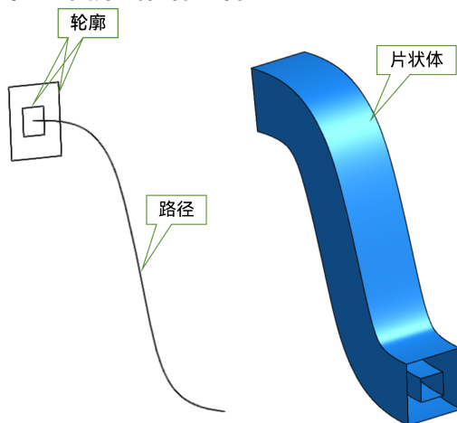
图 7-6 扫掠线框体组合
