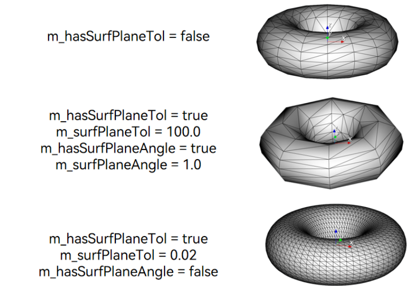
图 14-2 设置示例
