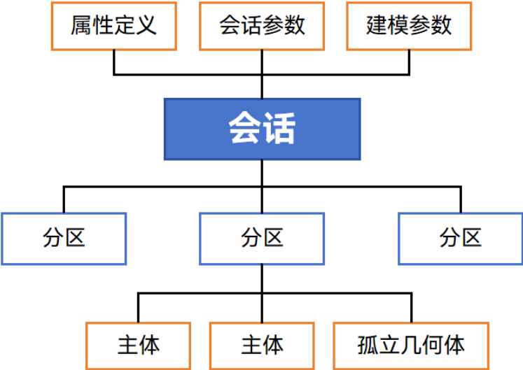
图 13-1 会话结构
