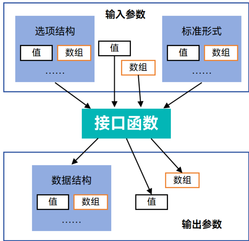
图 2-2 接口结构
