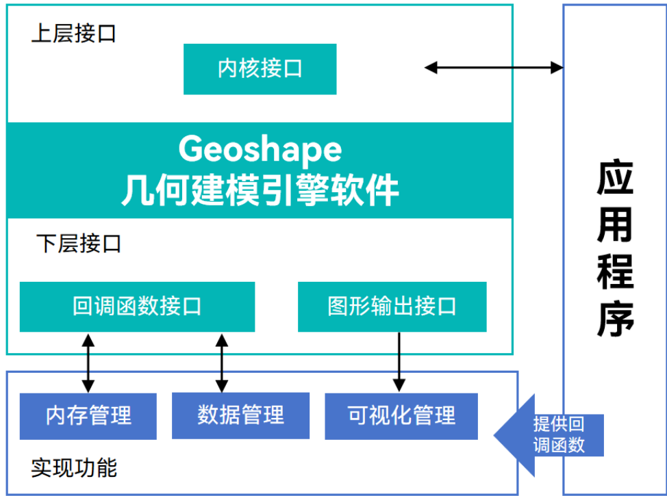
图 1-1 接口关系
