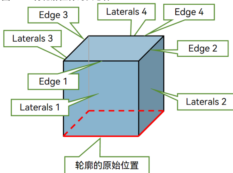
图 2-15 将轮廓拉伸为实体
