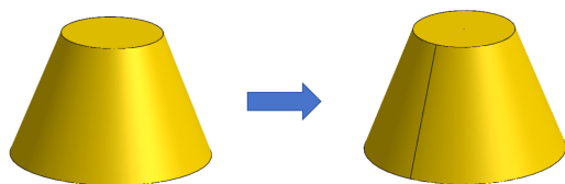
图 9-26 通过拆分拓扑创建的接缝
