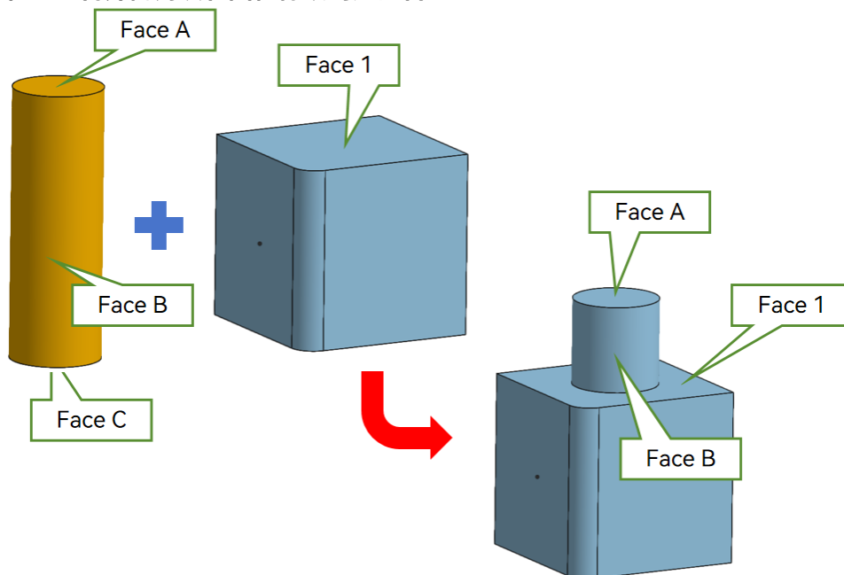
图 2-22 合并倒角块和圆柱体以创建凸台
