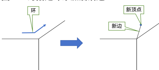
图 9-6 为指定环添加后沿边
