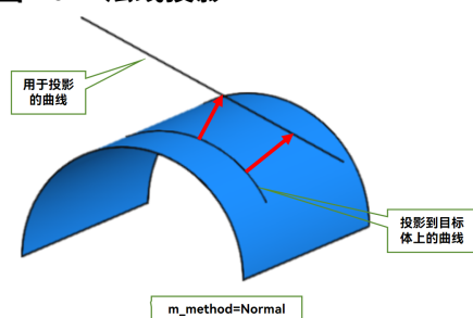
图 10-1 法线投影
