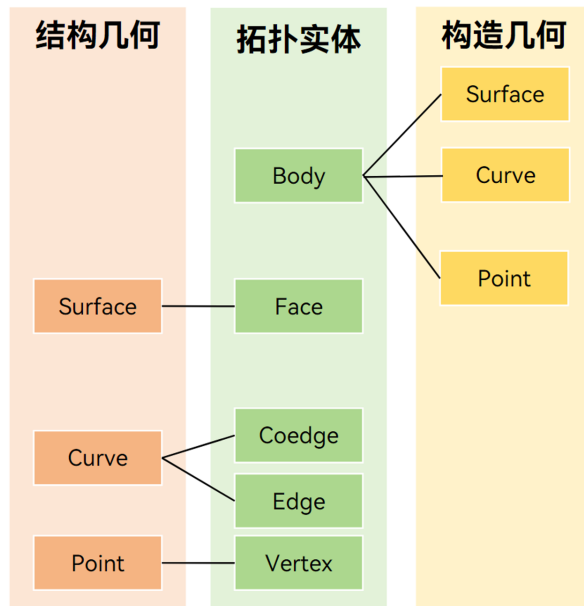
图 5-10 检查子主体上的系统属性时使用的实体层次结构
