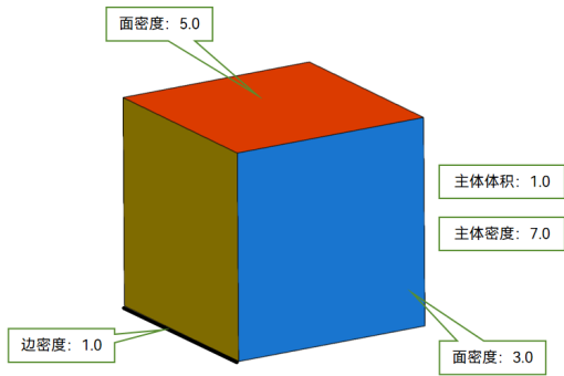
图 5-7 使用 m_lowerDimDensity 选项生成的 Mass 值
