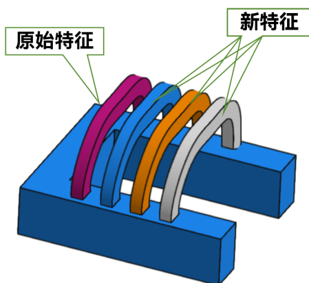
图 10-12 新实例位于与原始特征相同的面中
