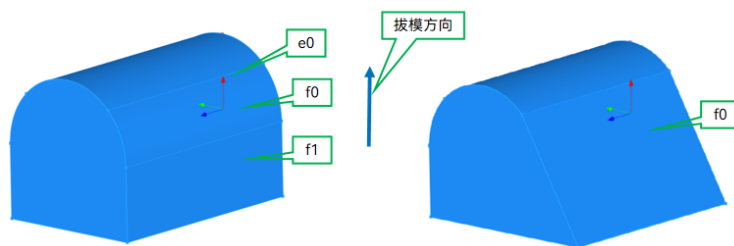
图 6-5 使用邻接面作为参考实体进行拔模
