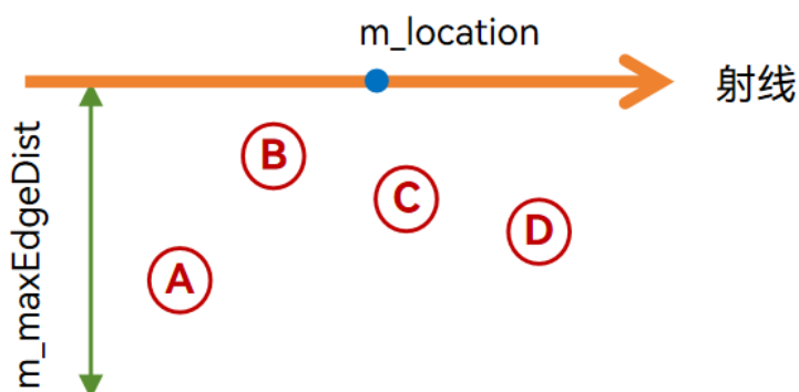
图 14-8 绝对位置排序
