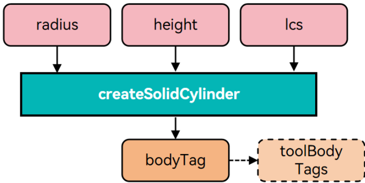
图 2-20 调用函数创建圆柱体
