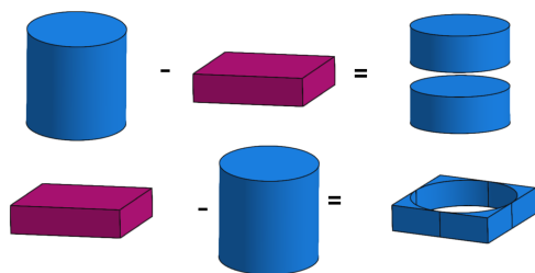
图 10-4 布尔减的目标体、工具体和结果体
