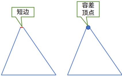
图 7-9 用容差顶点替换短边
