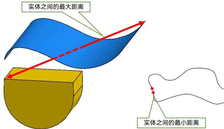
图 5-8 计算实体间的最大最小距离
