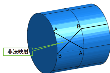
图 7-14 非法顶点映射示例二
