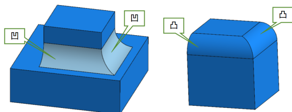
图 12-4 相同凸性倒角示例
