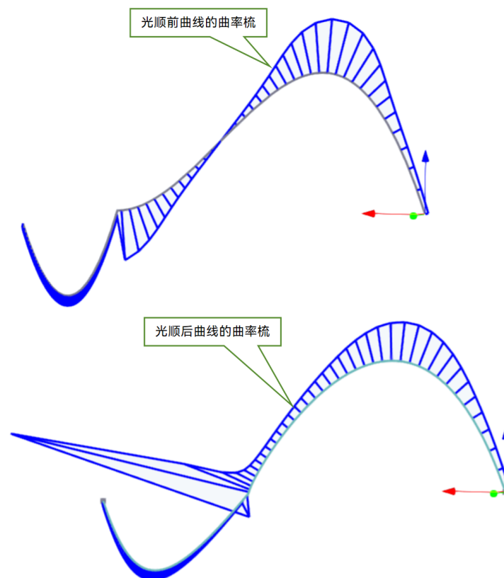
图 6-8 光顺前后曲线的曲率梳
