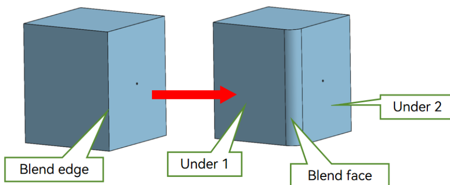
图 2-19 在一条边上添加倒角操作
