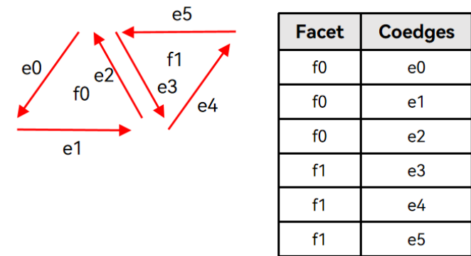
图 14-5 返回面片和半边的关系
