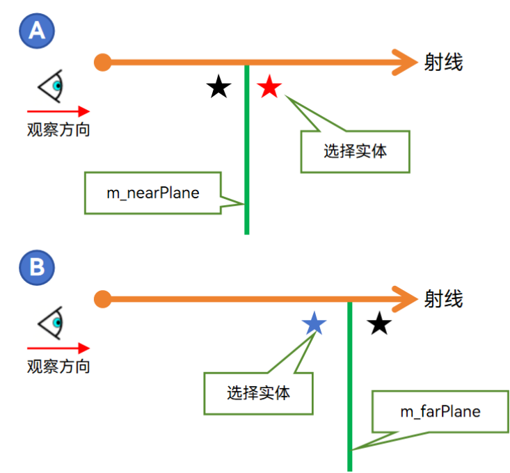
图 14-6 限制实体选择的范围
