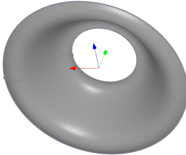
图 3-30 通过旋转 B 曲线创建 B 曲面
