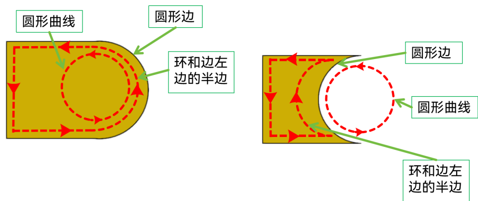
图 3-19 曲线、边、半边之间方向的关系
