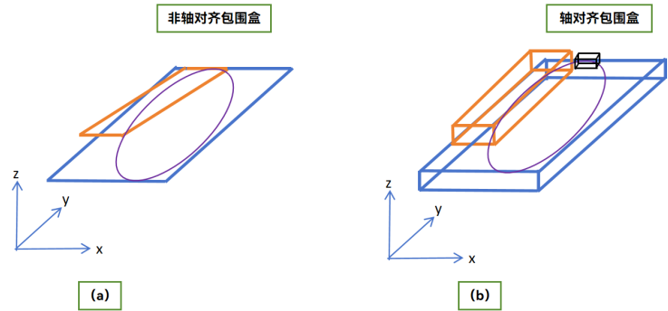
图 5-2 轴对齐和非轴对齐包围盒
