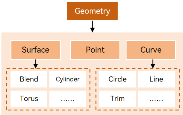
图 1-4 几何类
