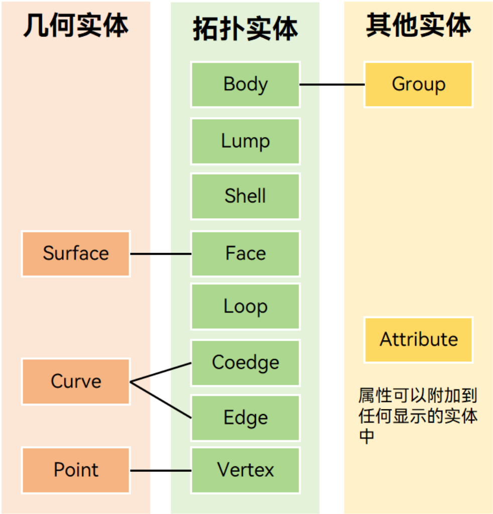
图 1-5 模型实体
