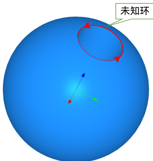
图 3-10 未知环示例
