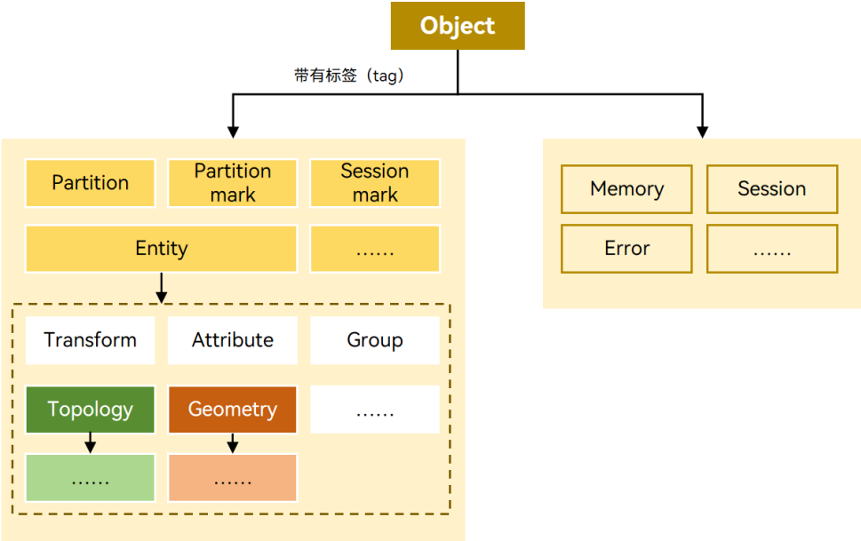
图 1-2 继承关系图
