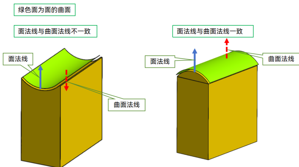
图 3-17 面方向标志
