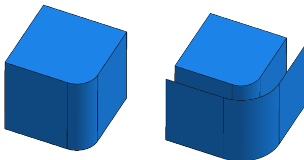
图 11-1 偏移示例
