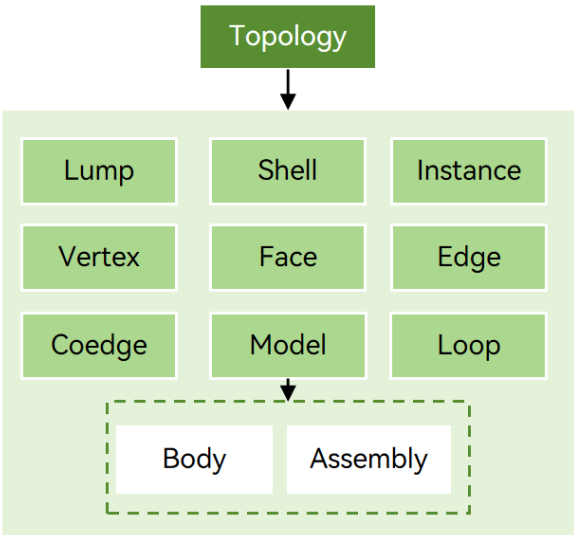
图 1-3 拓扑类
