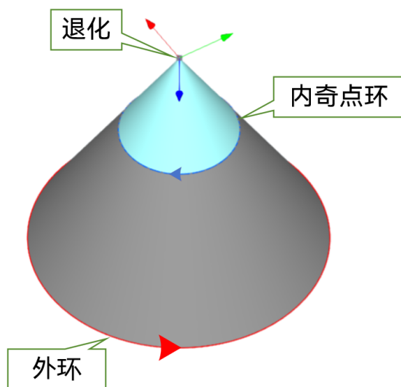
图 3-8 圆锥拓扑中的环
