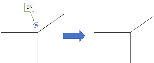
图 9-13 删除一个面上的一个孤立顶点和一个环
