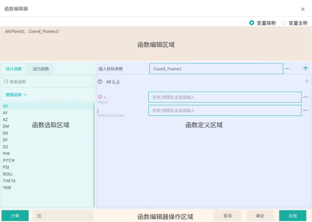
图 3-3 函数编辑器窗口
