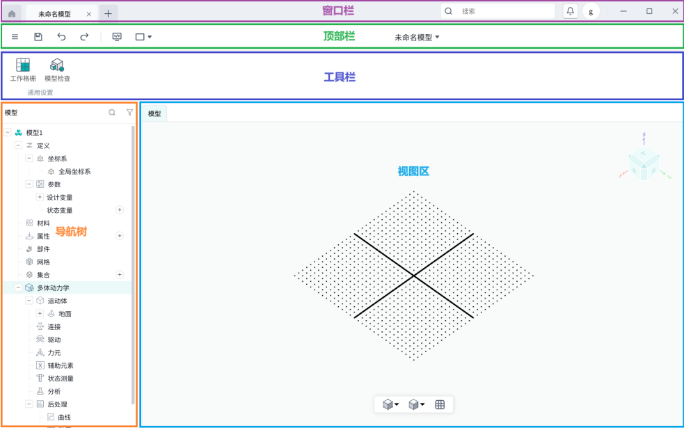
图 1-4 Workspace 窗口
