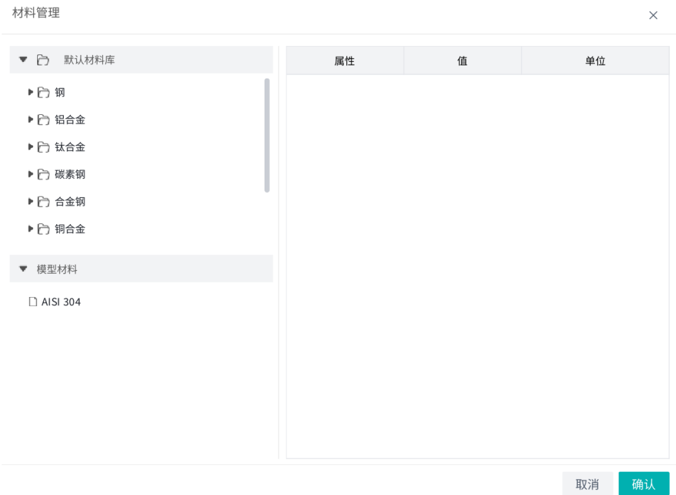
图 4-1 材料管理
