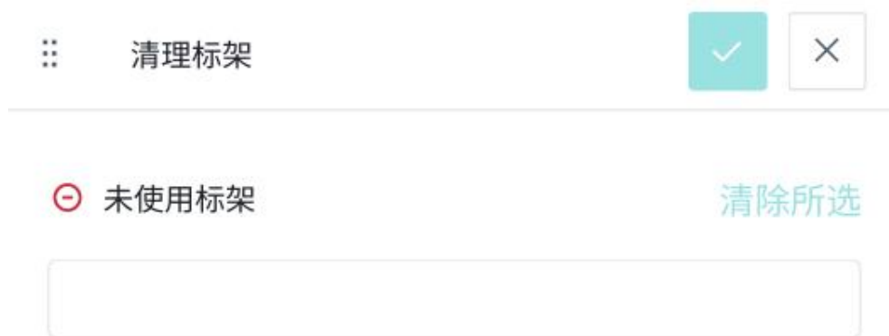
图 8-2 清理标架
