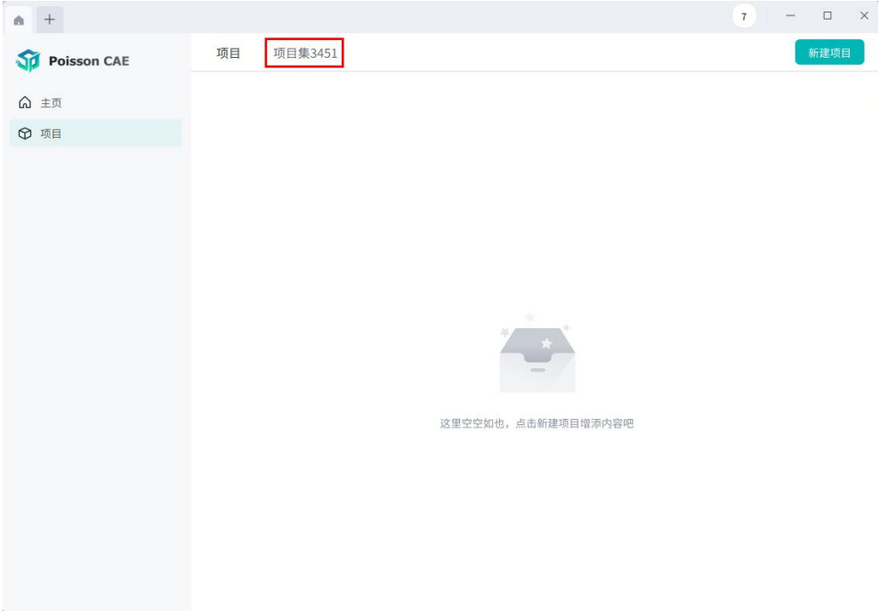
图 1-8 新建项目集
