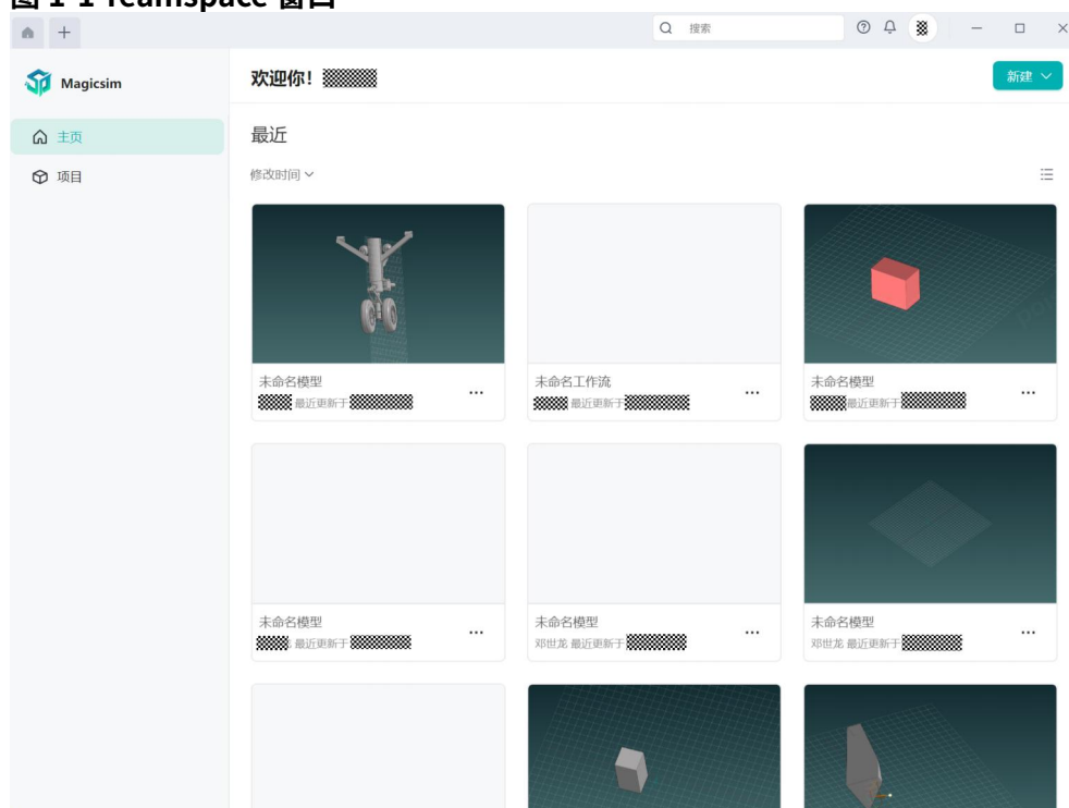
图 1-1 Teamspace 窗口
