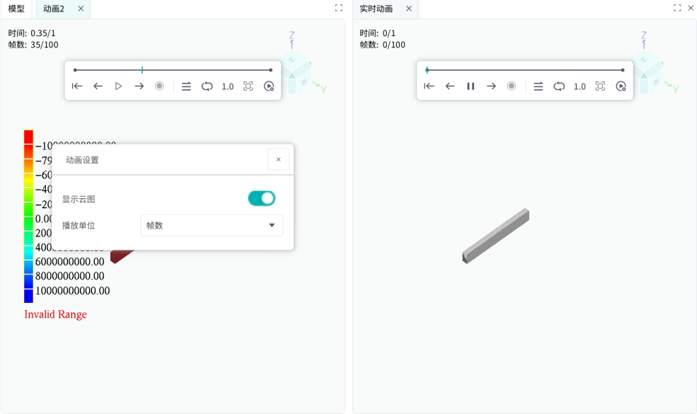
图 9-1 创建动画
