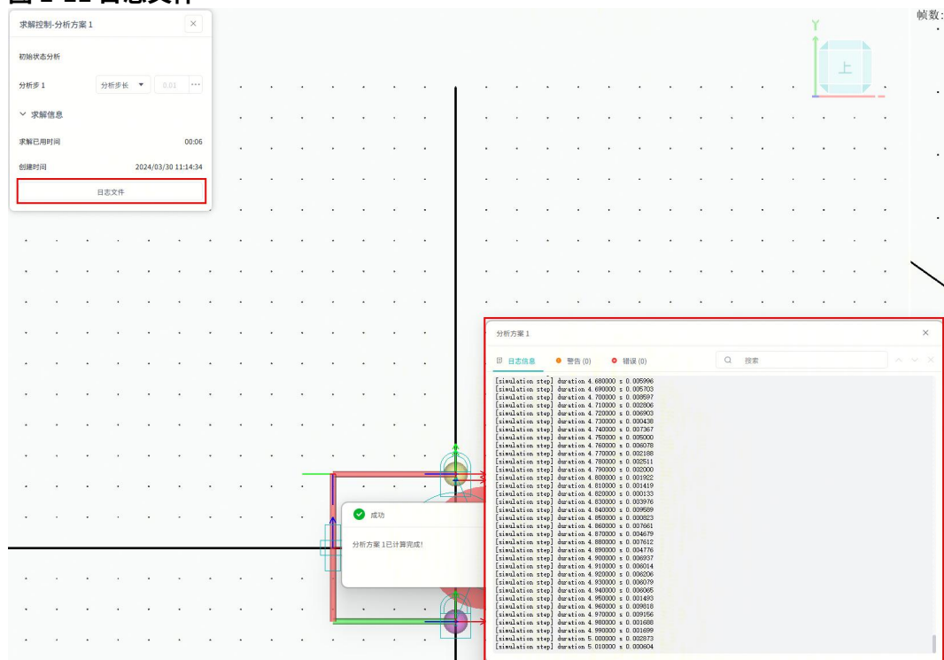
图 1-11 日志文件
