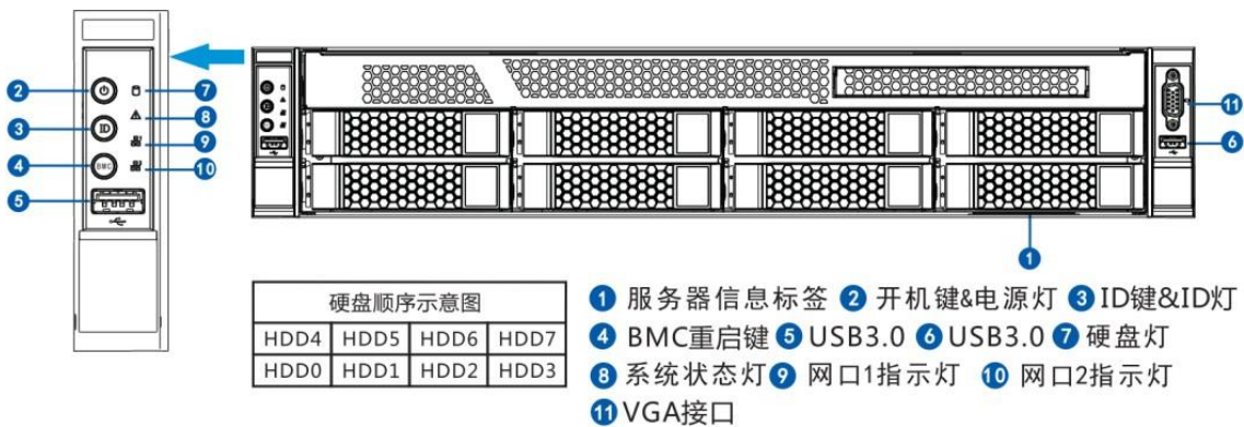
图 2-1 RT21-01 服务器前面板示意图
