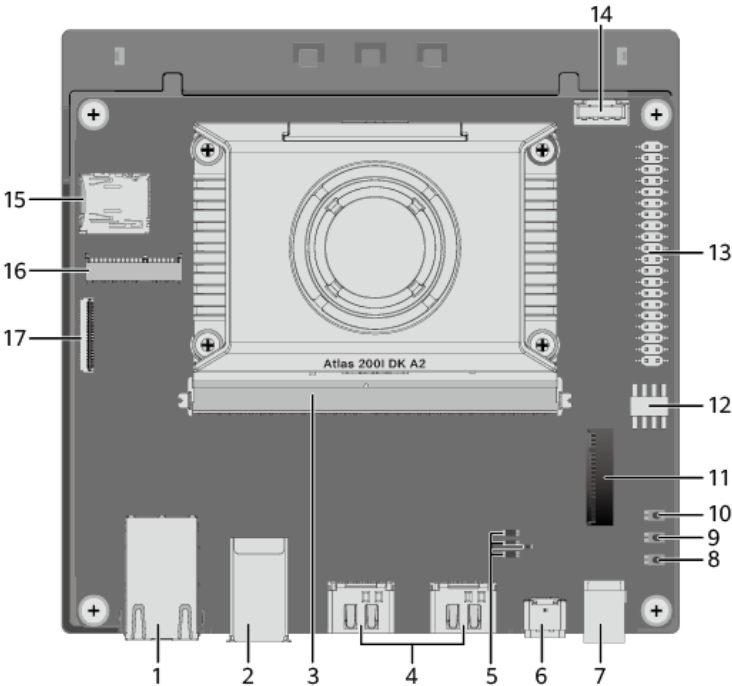
图 1-3 按键与接口说明
