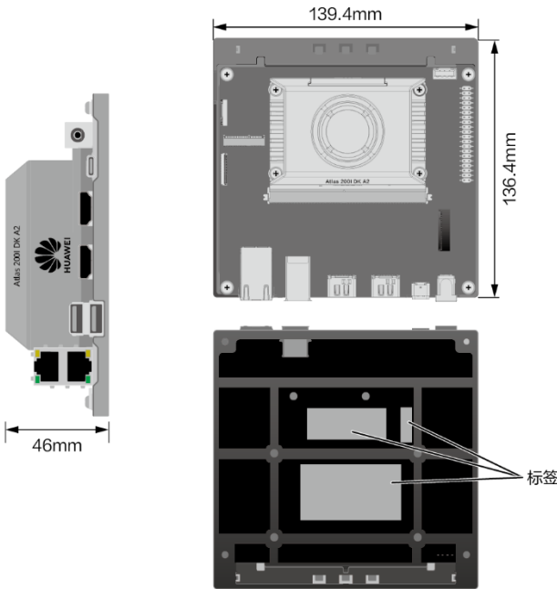
图 1-2 尺寸图（单位：mm）
