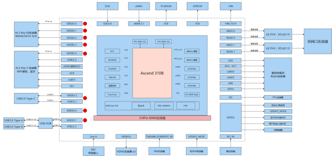
图 1-4 开发者套件系统框图
