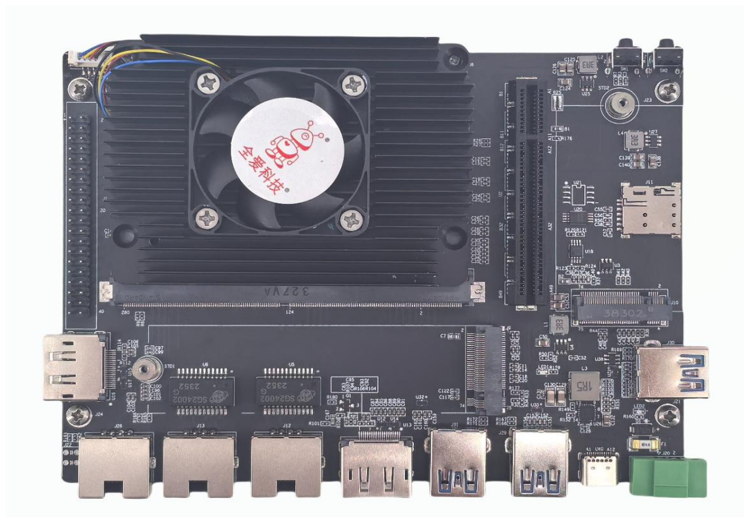
图 1.1 外观图
