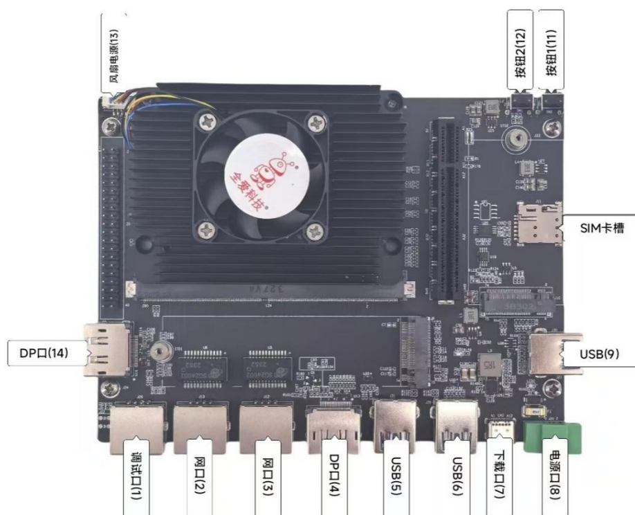
图 1.2 正面引脚图
