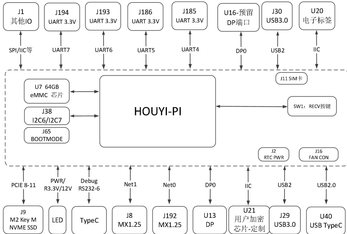
图 1.4 系统框图
