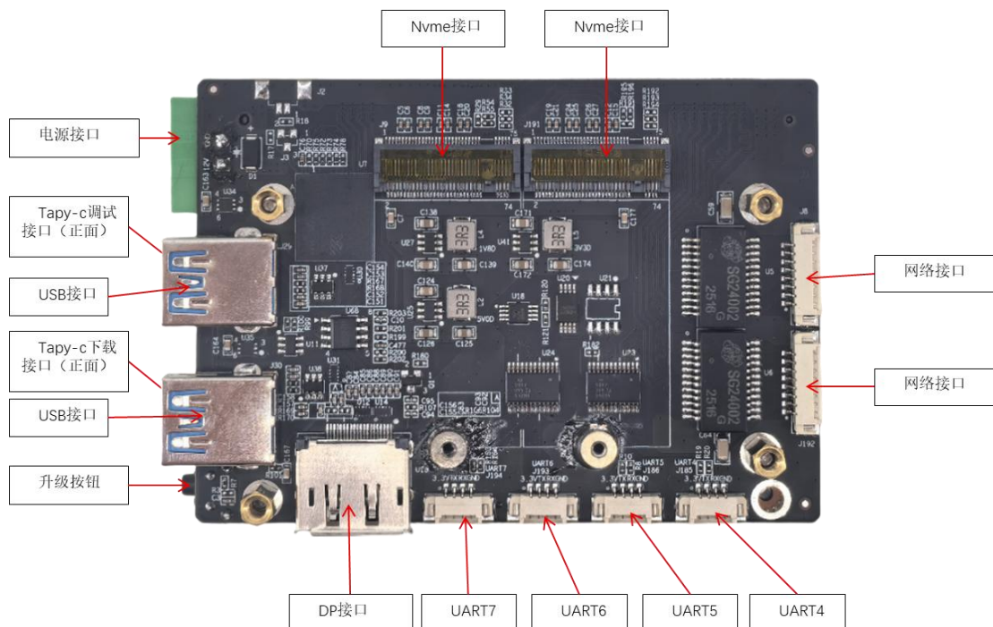
图 1.2 引脚图
